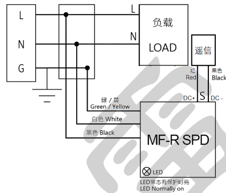
并联接法 Parallel Connection
